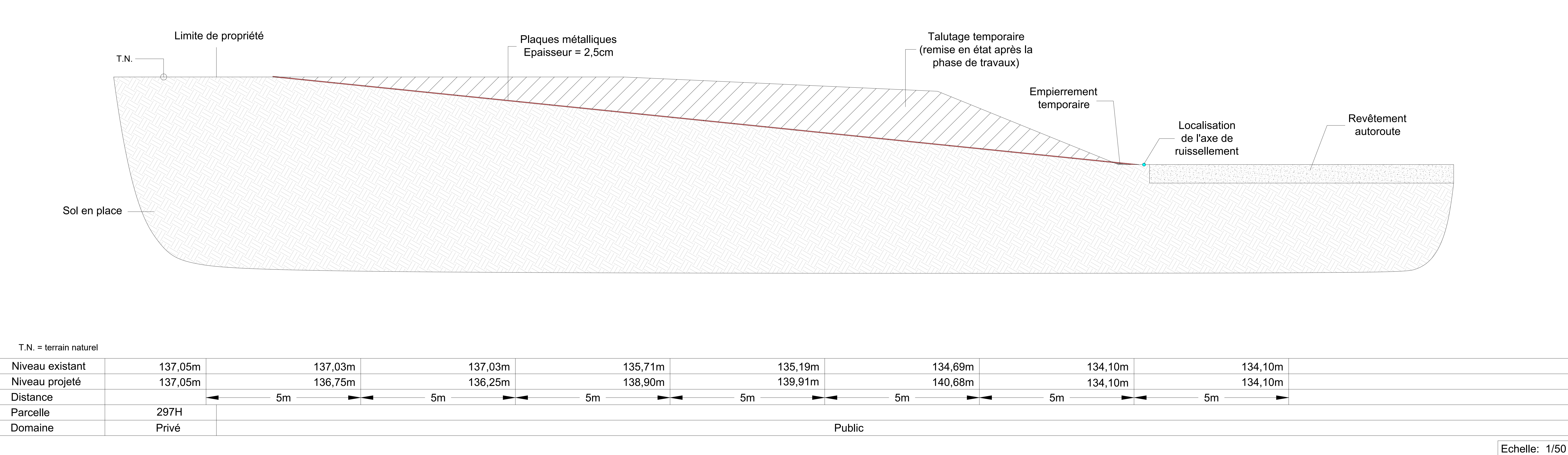
C03 - Coupe de principe de la création d'un accès temporaire en domaine privé vers les éoliennes n°2 et 3
