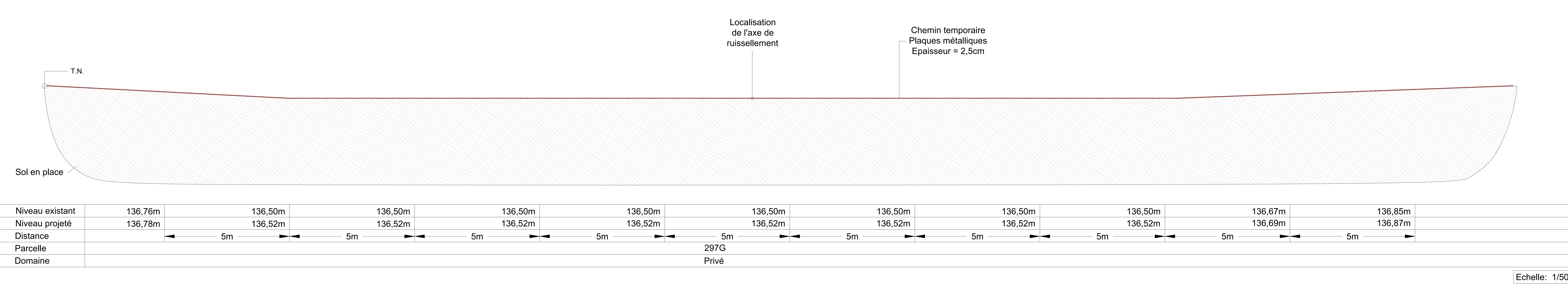
C03 - Coupe de principe de la création d'un accès temporaire en domaine privé vers les éoliennes n°2 et 3
