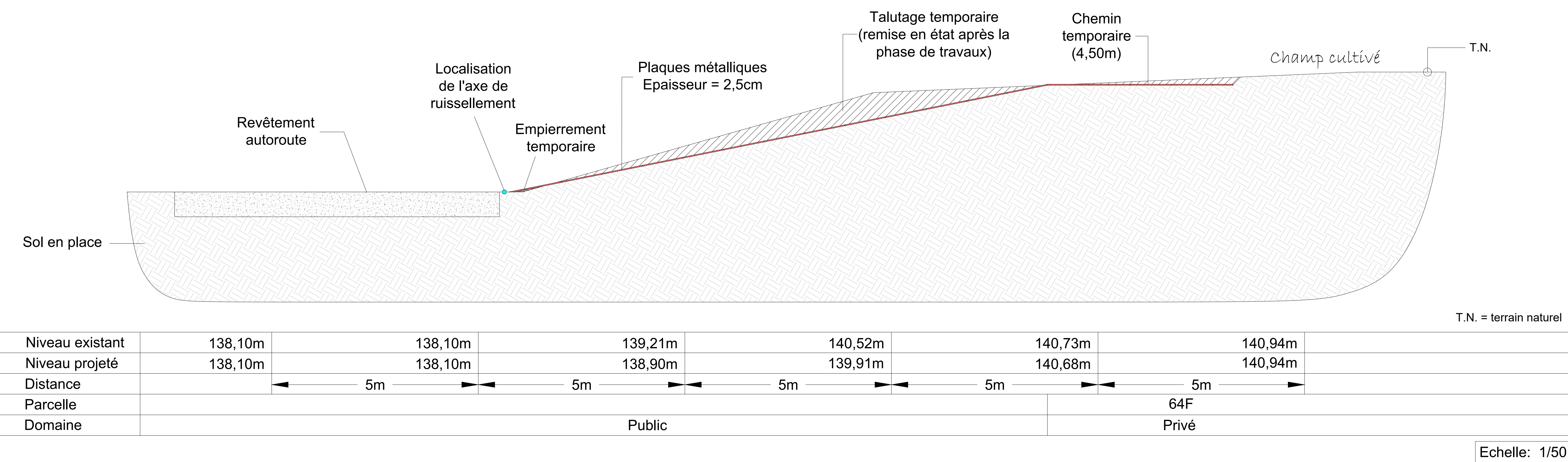
C02 - Coupe de principe de la création d'un accès temporaire en domaine public vers les éoliennes n°2 et 3
